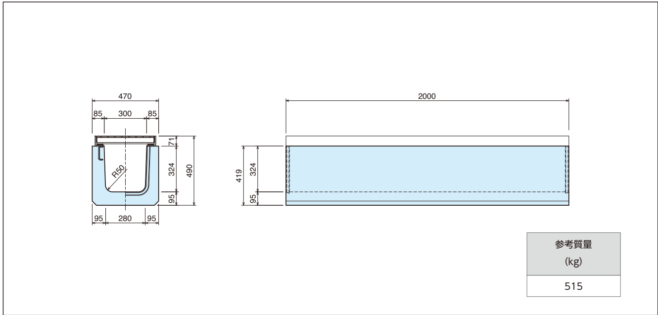
[形状図 (JIS規格 道路側溝 (3種) 300A対応タイプ)]
