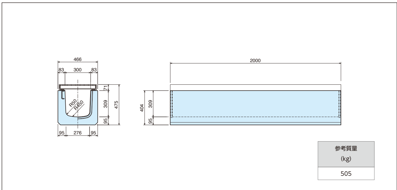
[形状図 (浸透側溝 EX 300×300×2000対応タイプ)]
