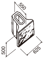
〈500B型〉 大谷石189kg
