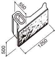
〈500B型〉 大谷石189kg
