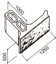
〈1000A型〉 大谷石414kg
