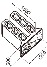
〈1500W型〉 大谷石807kg
