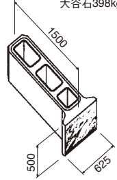
〈N1500B型〉 大谷石398kg
