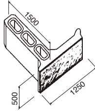
〈1500A型〉 大谷石527kg
