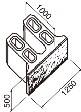
〈1000W型〉 大谷石584kg
