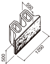
〈500W型〉 大谷石393kg
