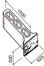
〈1500W型〉 大谷石807kg
