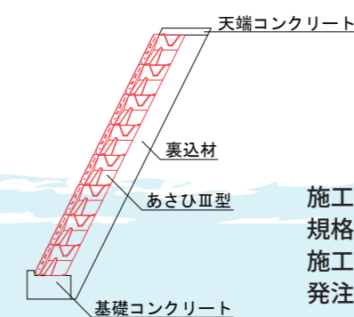
標準断面図
